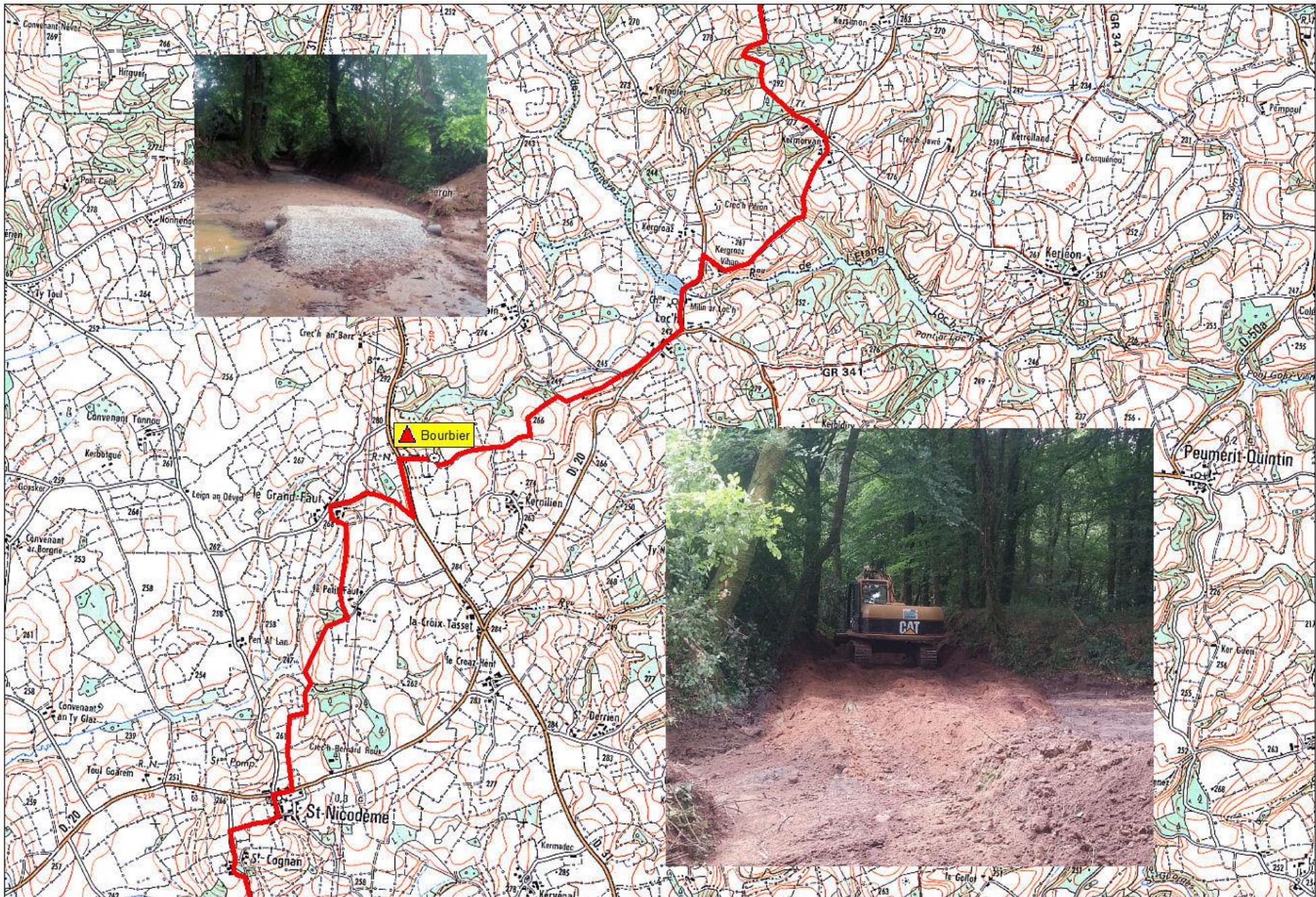
Chantier du 29/06/2016 à Peumerit-Quintin : assainissement d'un bourbier
